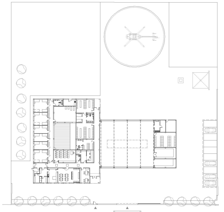
CONCURS PER LA NOVA CONSTRUCCIÓ DEL PARC DE BOMBERS DE VALLS GISA 2007. 2n PREMI
